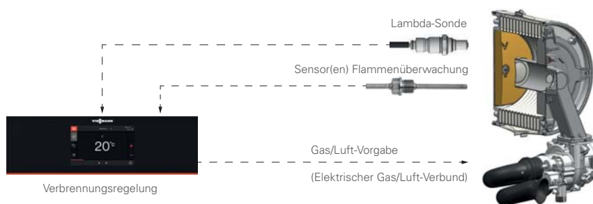
Sensorgeführte elektronische Verbrennungsregelung mit Lambda-Sonde
